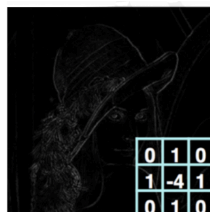
Edge Detect
